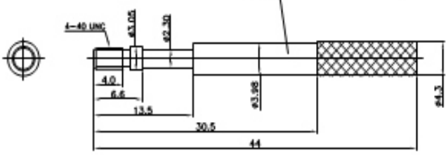
Long BOLT
